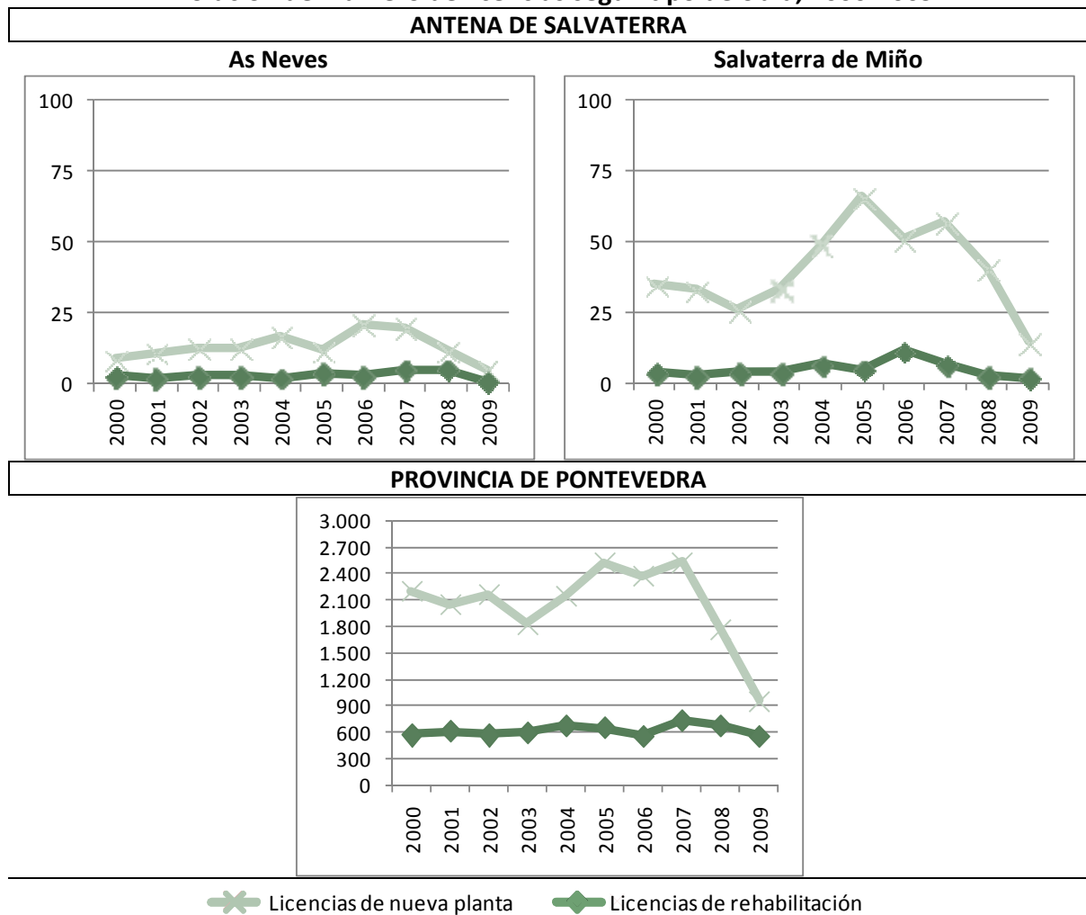
Figura 21 Evolución del número de licencias según tipo de obra, 2000-2009
